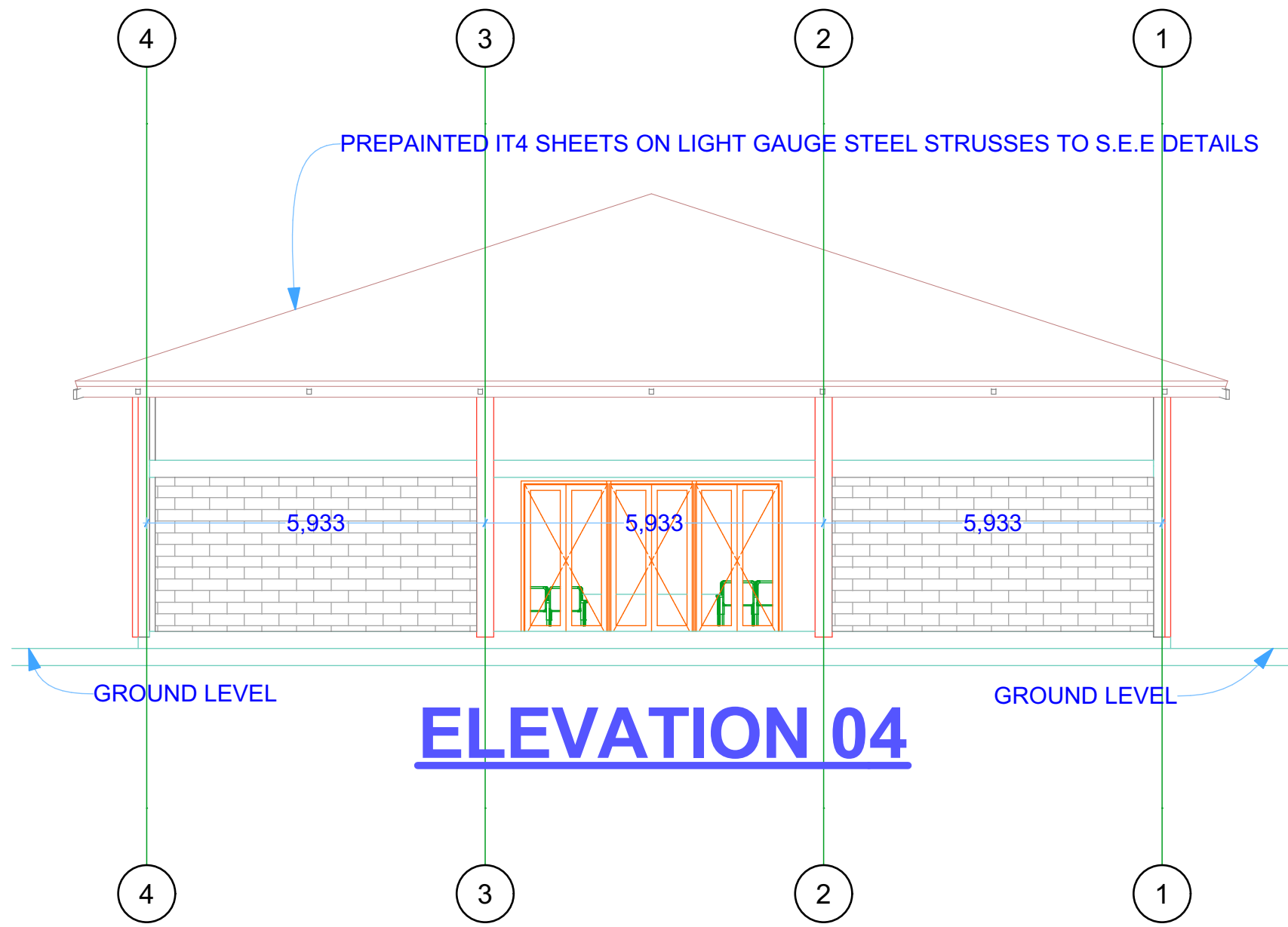
E-04 Elevation 1:100
