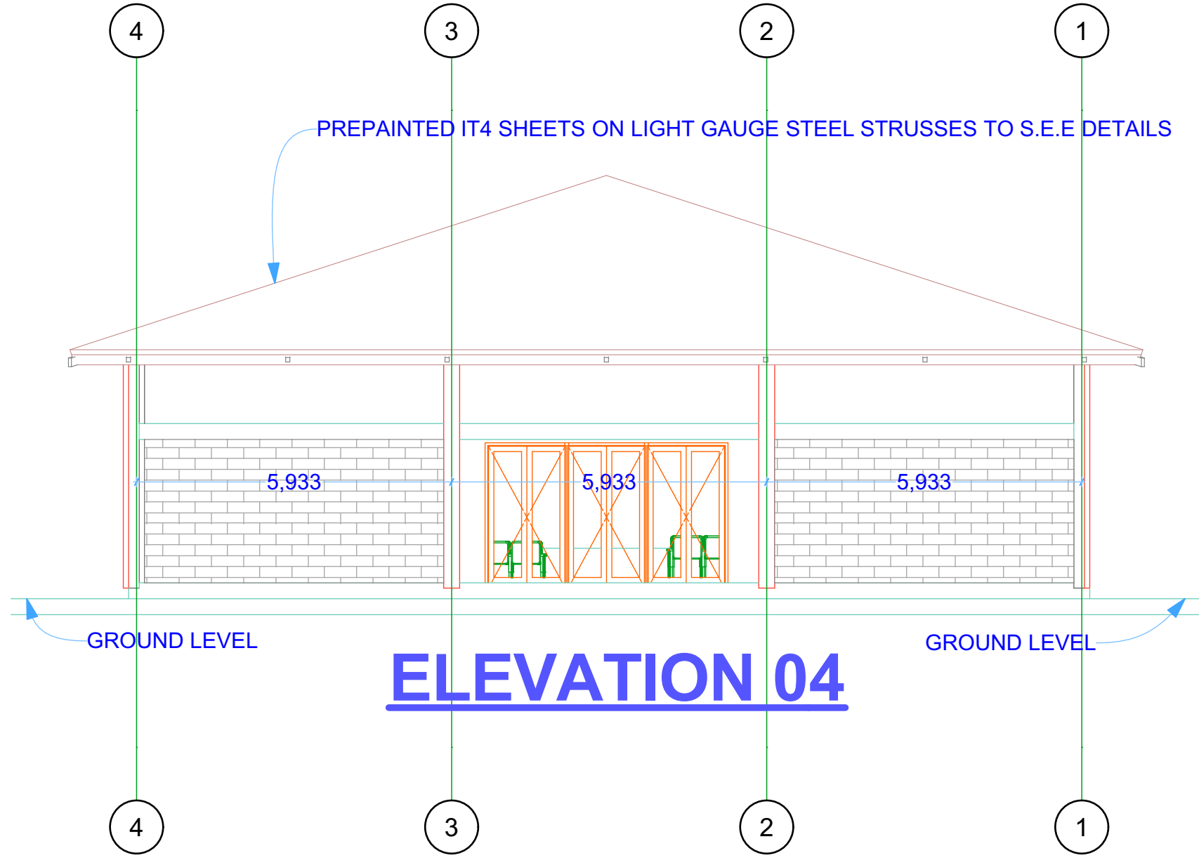
E-04 Elevation 1:100
