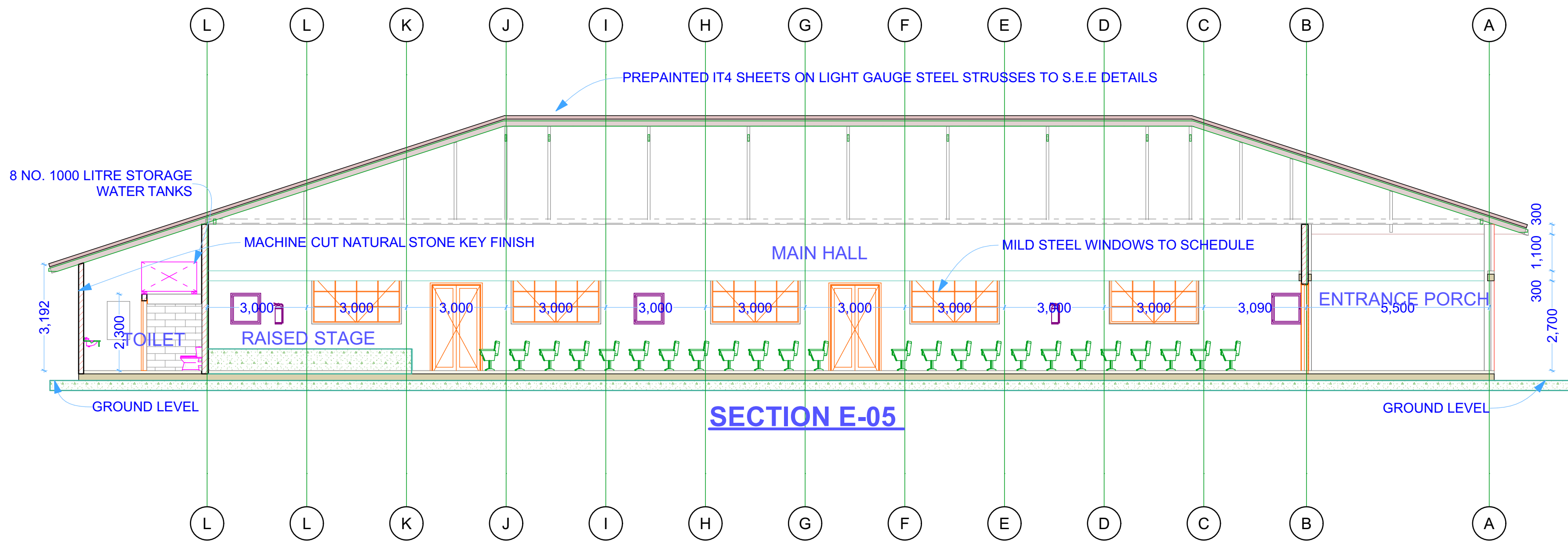
E-05 Elevation 1:100
