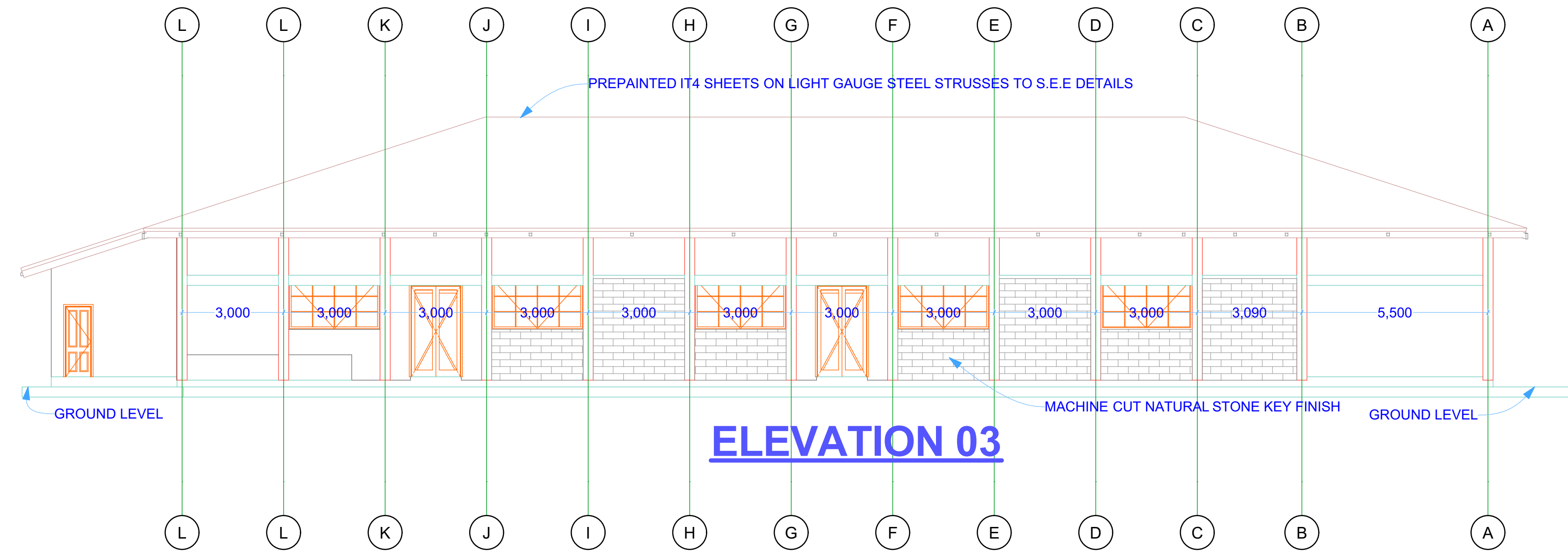
E-03 Elevation 1:100
